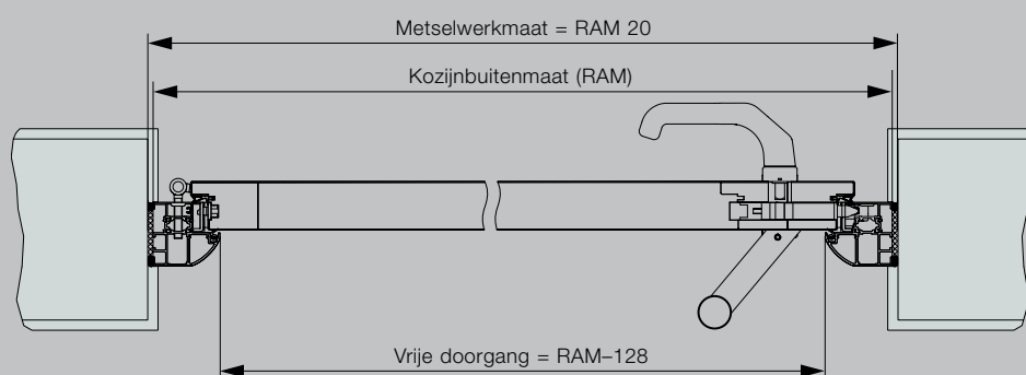
Verbreidingsprofiel 25 mm
