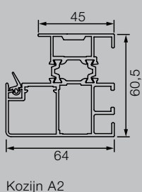
Kozijn A2
