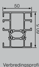
Verbreidingsprofiel 50 mm
