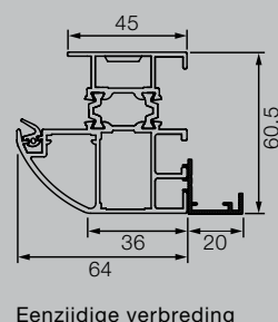
Eenzijdige verbreding
