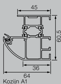
Kozijn A1
