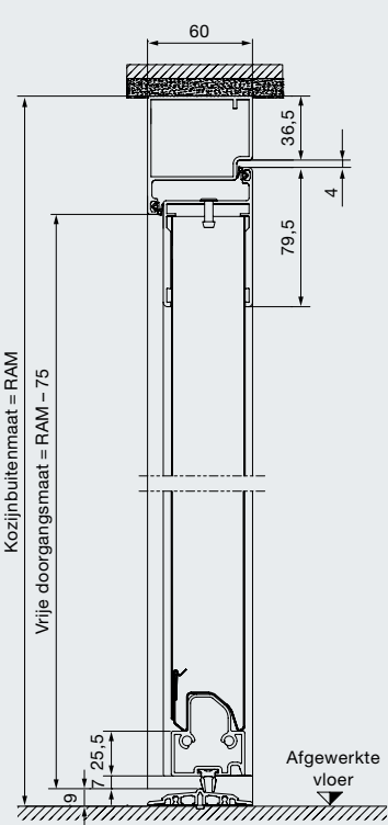
Verticale doorsnede NT 60-2
