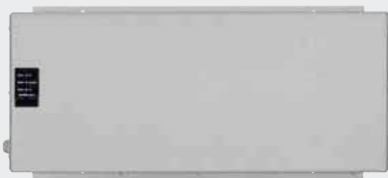
USV-installatie Ter overbrugging van spanningsuitvallen tot max. 4 uur, veiligheidsvoorzieningen, signaallichten etc. blijven werken, LED-statusindicatie, automatische accutest, overspanningsfilter, afmetingen: 560 x 235 x 260 mm (B x H x D), Beschermingsgraad: IP 20
