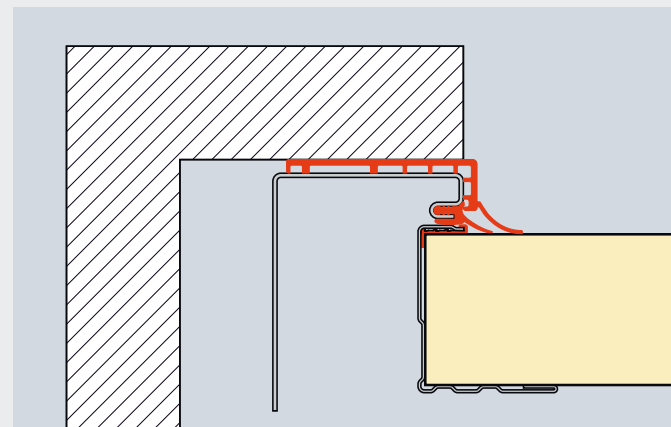
Zijdelingse aanslag met ThermoFrame
