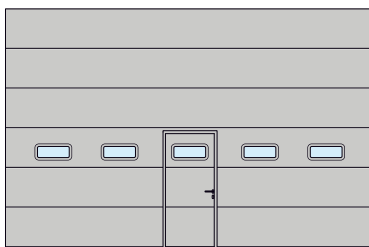
SPU F42 Panelen met sandwichvensters type A Loopdeurpositie midden
