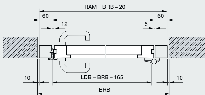
Inbouw in de opening
