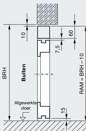
Inbouw in de opening
