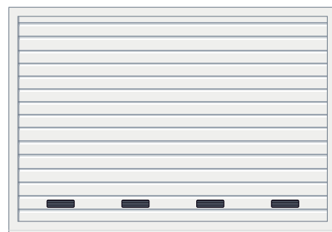
Motief 480 , paneelvulling met ventilatieroosters. Ventilatie-doorlaat: 40 cm 2 /rooster
