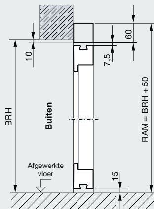
Inbouw achter de opening
