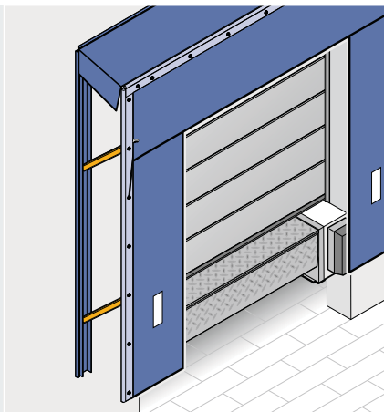
Linkarm constructie
