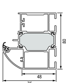
Kozijn A3
