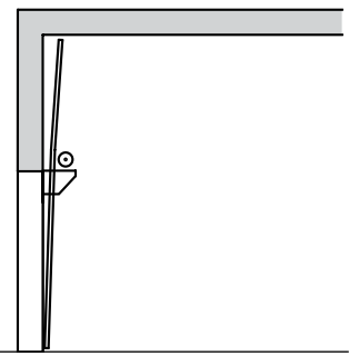
Beslagtype VU Met onderliggende veeras
