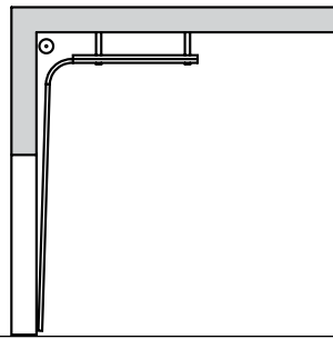
Beslagtype H Verhoogd looprailbeslag
