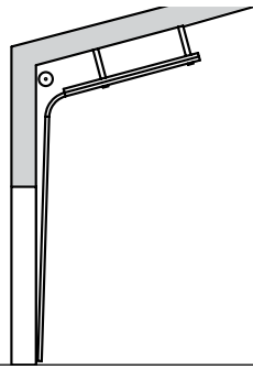
Beslagtype HD Daklijnvloegend
