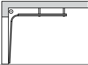
Beslagtype N Normaal beslag
