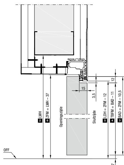
Verticale doorsnede type RI met reverse openend deurblad
