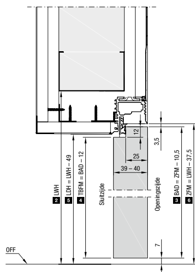
Verticale doorsnede type NA met normaal openend deurblad
