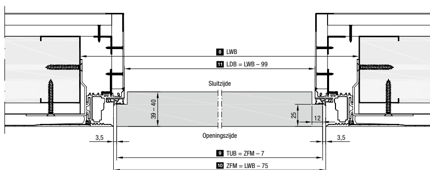
Horizontale doorsnede type NA met normaal openend deurblad
