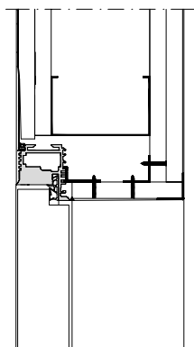
Verticale doorsnede normaal naar buiten openend (type NA)
