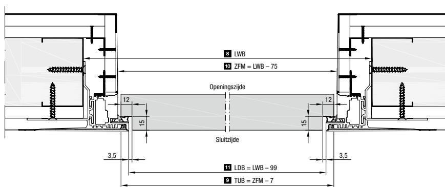
Horizontale doorsnede type RI met reverse openend deurblad
