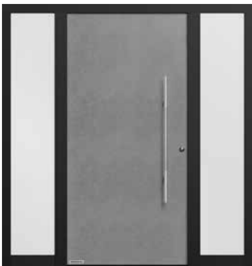
Aluminium voordeur ThermoSafe motief 860 Deurblad in Decoral cement, deurkozijn in gitzwart RAL 9005 fijnstructuur, roestvrijstalen handgreep HOE 700, zijdelen met figuurglas Satinato
