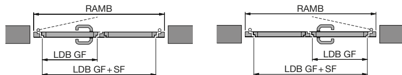
DIN rechts, naar buiten openend
