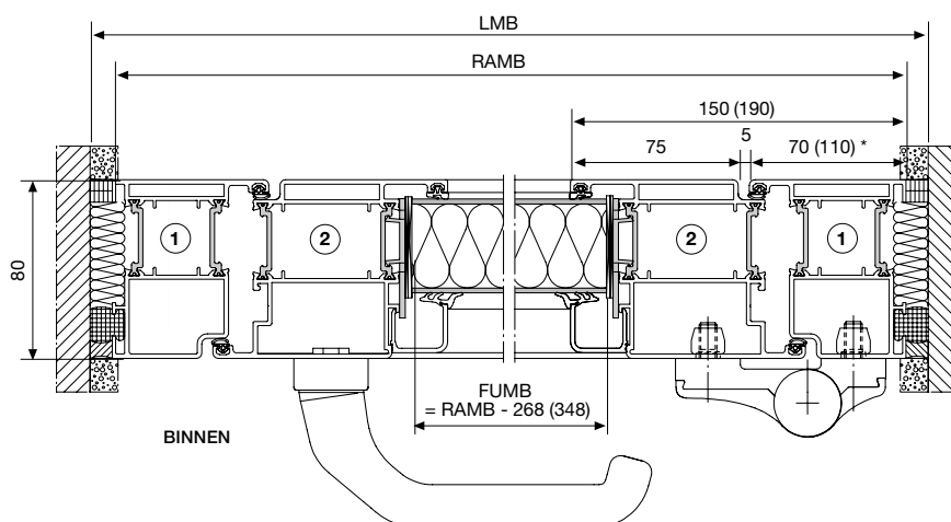
Horizontale doorsnede
