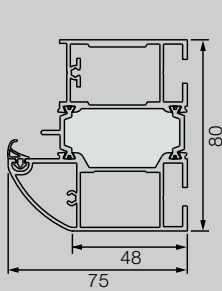
Kozijn A3
