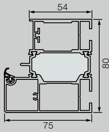
Kozijn A4
