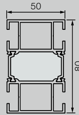
Verbreidingsprofiel 50 mm
